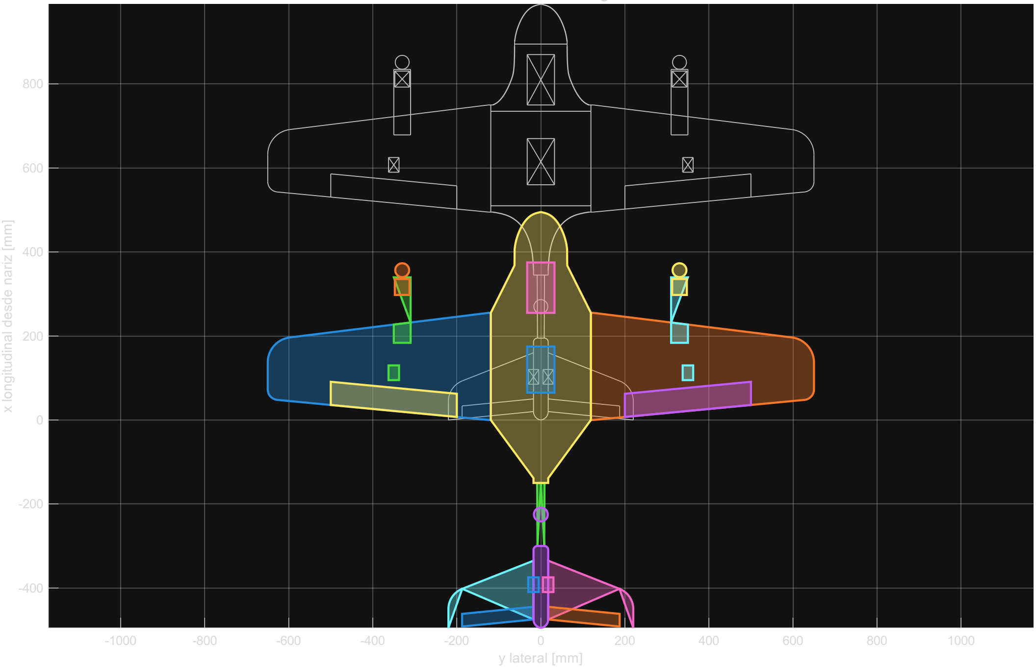
Partes DXF sobre silueta general
